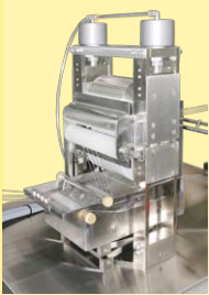
foulard de impregnación con tina calentada
