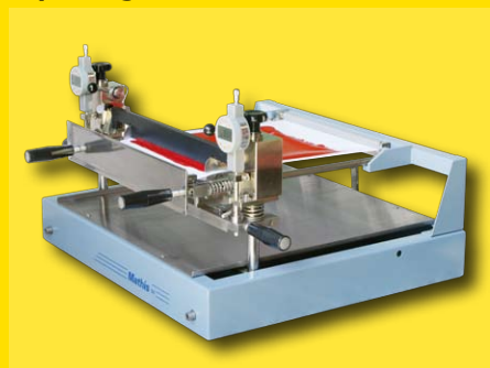
Equipamento de laboratório para espatulagem em papel - SVA-B (opcional: com pré-secagem IR)
